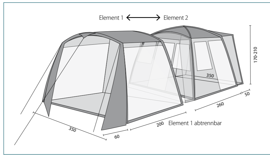
Rückwand mit Hochentlüftung
