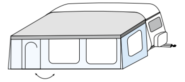
Türe links, 2 große Fenster rechts
